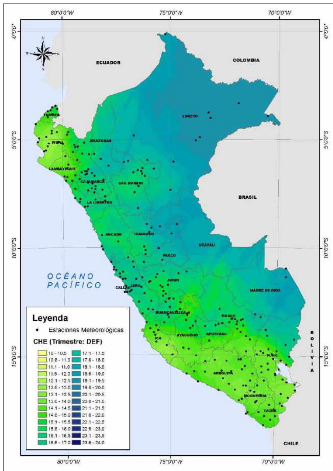
Figura 2. Mapa del Contenido de Humedad Teórico - Trimestre Dic/Ene/Feb
